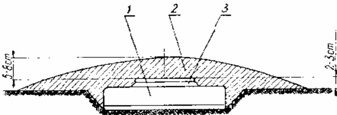
Rys. 46 Sposób ustawienia miny ppanc w gruncie twardym.
