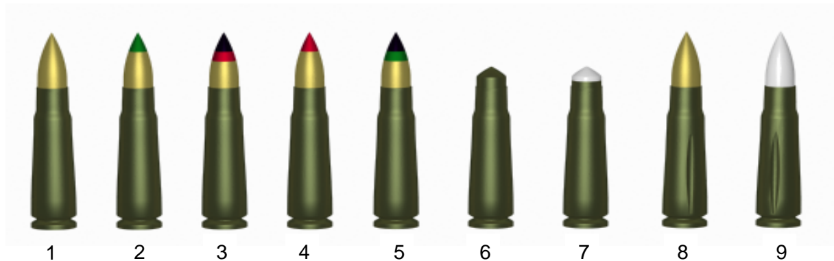
Rys. 32. 7,62mm naboje wz 1943: 1 – z pociskiem zwykłym PS, 2 – z pociskiem smugowym T- 45, 3 – z pociskiem przeciwpancerno – zapalającym BZ, 4 – z pociskiem zapalającym Z, 5 – z pociskiem o zmniejszonej prędkości US, 6 – nabój ślepy, 7 – nabój miotający UNM, 8 – nabój szkolny, 9 – nabój treningowy.
