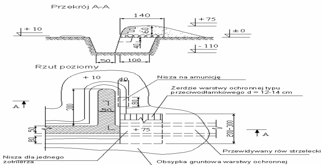
Rys. 38. Okop do strzelania z rpgpanc z ukryciem dla jednego żołnierza.
