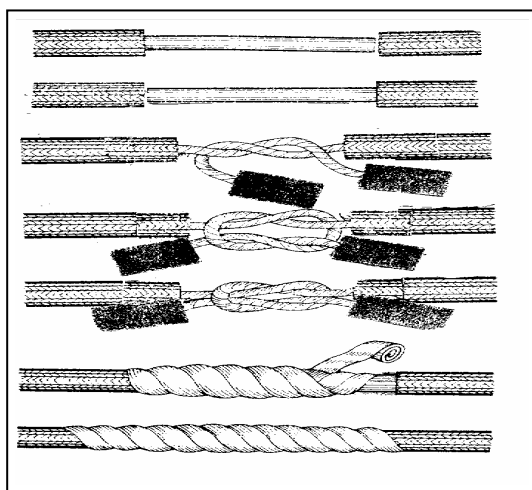
Rys. 35. Wykonanie złącza na linii przewodowej PKL 1x2*: a, b, c, d, e, f, - kolejne fazy wykonywania poszczególnych czynności *PKL 1x2 – Połowy Kabel Lekki.
