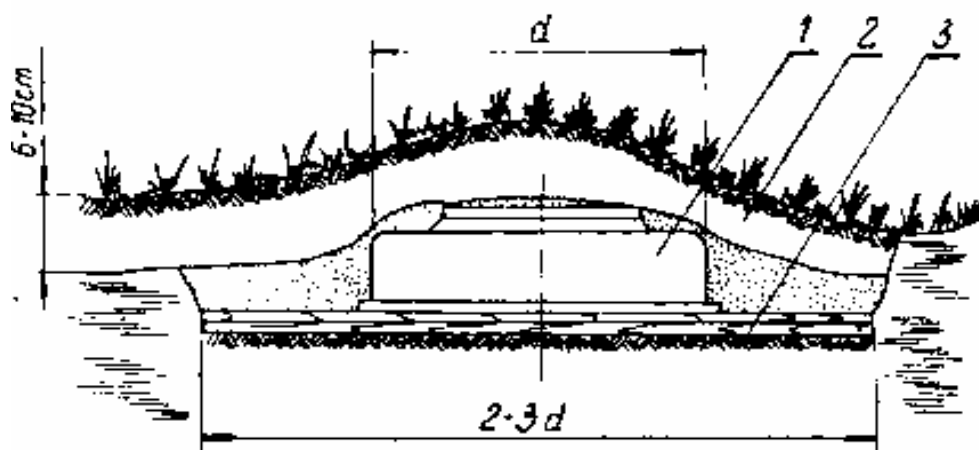
Rys. 47. Sposób ustawienia miny ppanc w terenie podmokłym lub błotnistym 1 – mina, 2 – warstwa maskująca minę, 3 – podkładki z desek. Źródło: opracowanie własne
