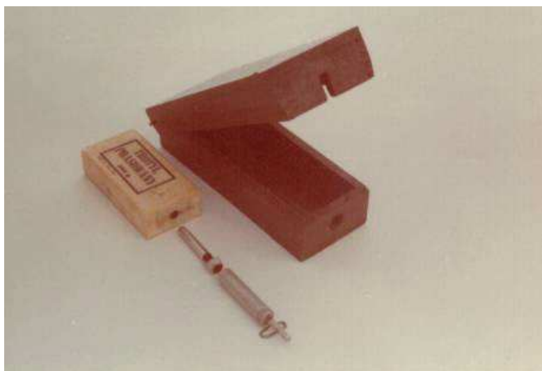
Fot. 105. Mina PMD-6M.
