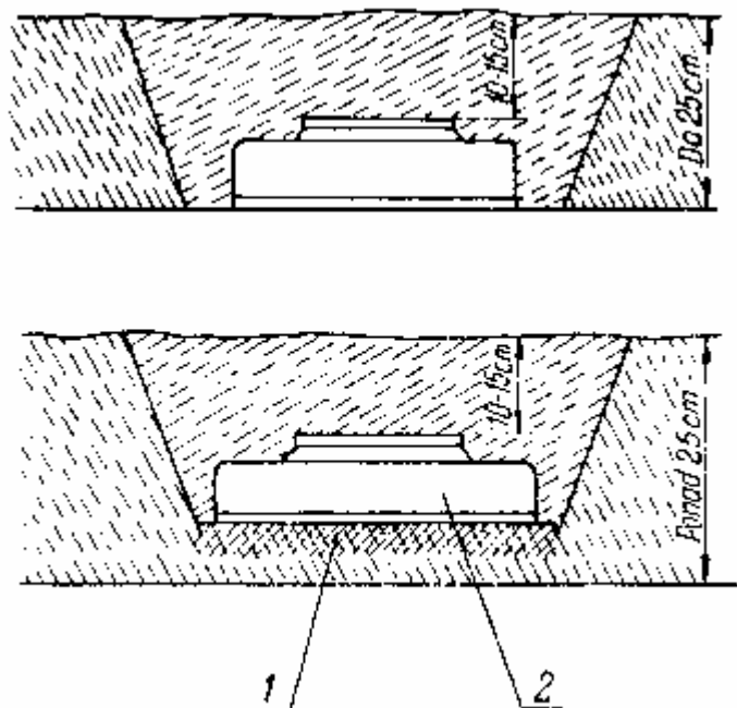
Rys. 44. Sposób ustawienia miny ppanc zamaskowanej śniegiem.
