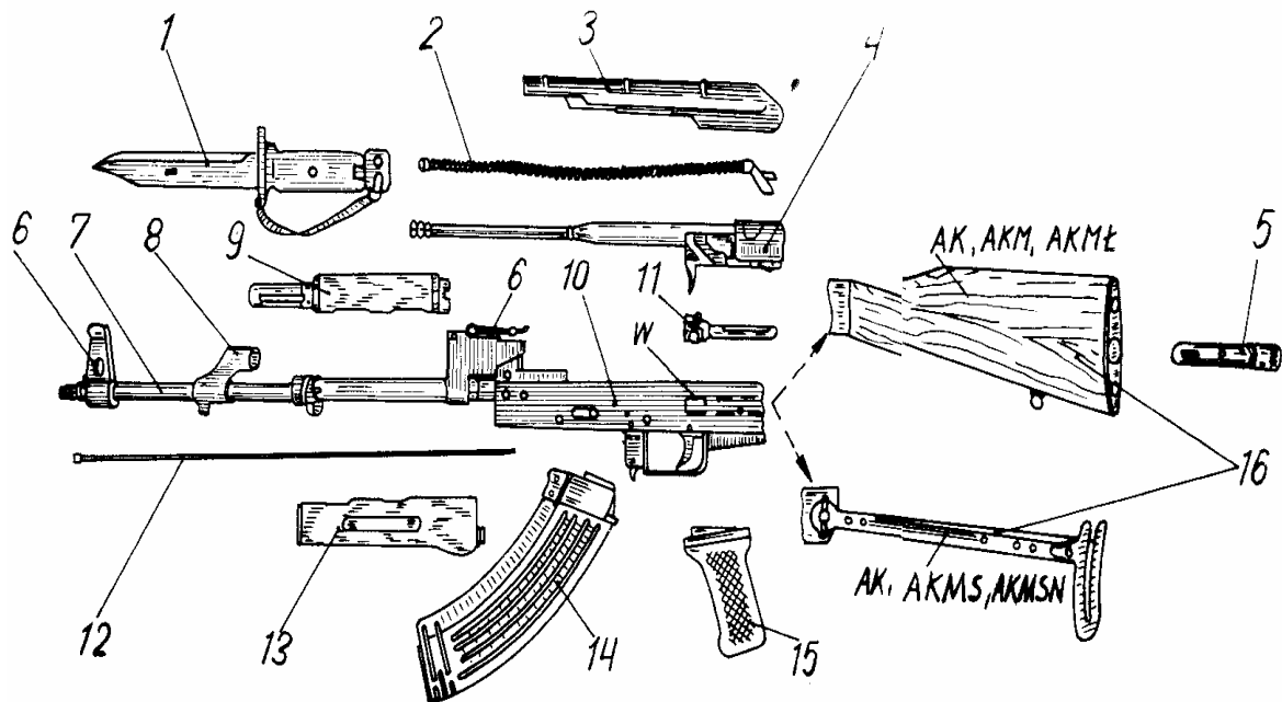
Rys. 28. Zasadnicze zespoły i części karabinków AKM (AKMŁ), AKMS (AKMSN) i AK:
