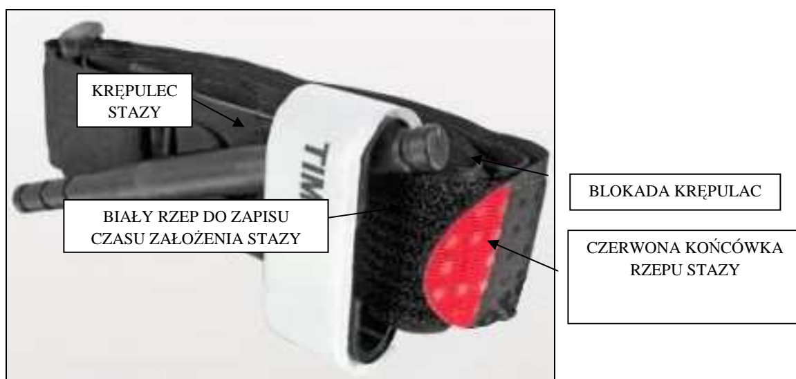
Fot. 70. Opis elementów stazy taktycznej typu CAT.
