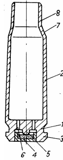
Rys. 31. Łuska naboju pośredniego 1 – dno, 2 – tułów, 3 – kryza, 4 – spłonka, 5 – kowadełko, 6 – otwory ogniowe, 7 – stożek przejściowy, 8 – szyjka łuski. Źródło: opracowanie własne
