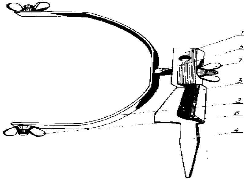
Rys. 59. Urządzenie do ustawiania miny MON-100.
