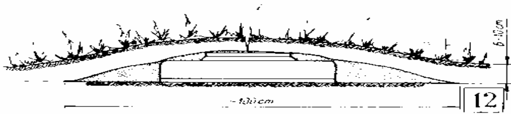
Rys.42. Sposób ustawienia miny ppanc zamaskowanej darnią.
