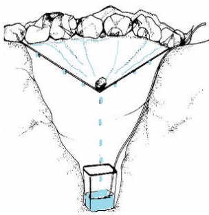
Rys. 21. Sposób wykonania destylarki słonecznej.
