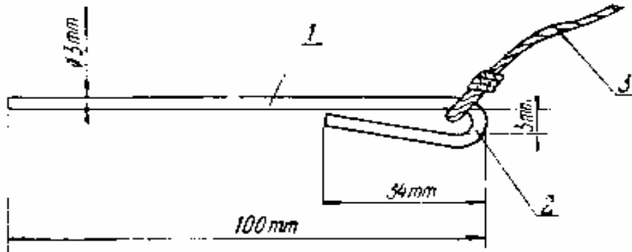
Rys. 55. Podpórka zabezpieczająca miny PMD-6.
