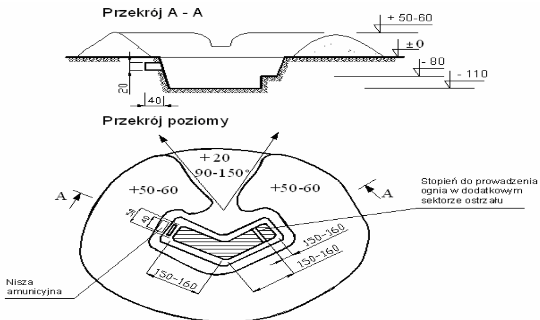
Rys. 37. Okop do strzelania z karabinu maszynowego.
